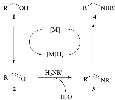
图式 1 借氢策略
